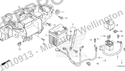
C-37 Bateria
