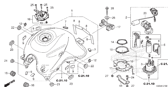
C-21 Tanque de Combustível • Bomba de Combustível (ESD/EX)
