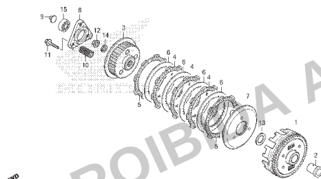
M-8 Embreagem
