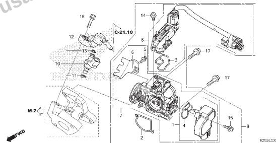
M-23 Corpo do Acelerador • Injetor de Combustível (ESD/EX)
