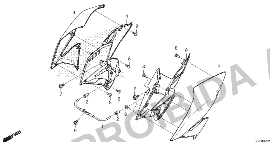
C-22.1 Carenagem (EX)
