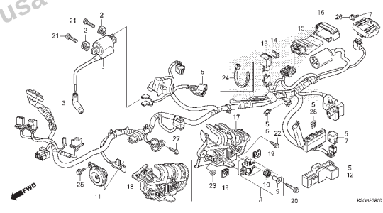
C-38 Fiação Principal
