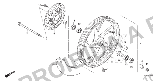
C-14.40 Roda Dianteira (ESD/EX)
