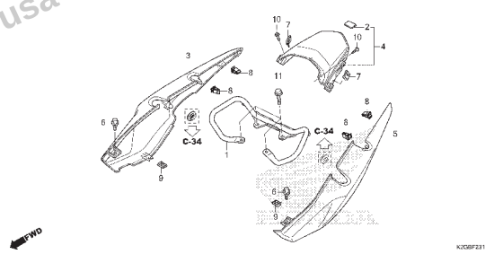
C-23.10 Rabeta (ES/ESD)
