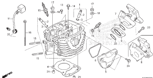
M-5 Cilindro
