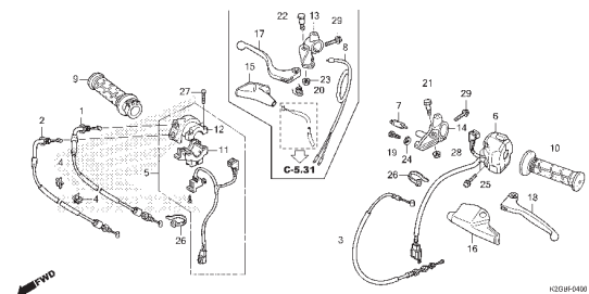
C-5.31 Cabo do Freio (ES)
